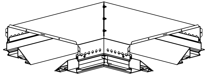
Corner Unit ALS-EL-H06-043-MB Feed Corner ALS-LF-H06-043-MB
